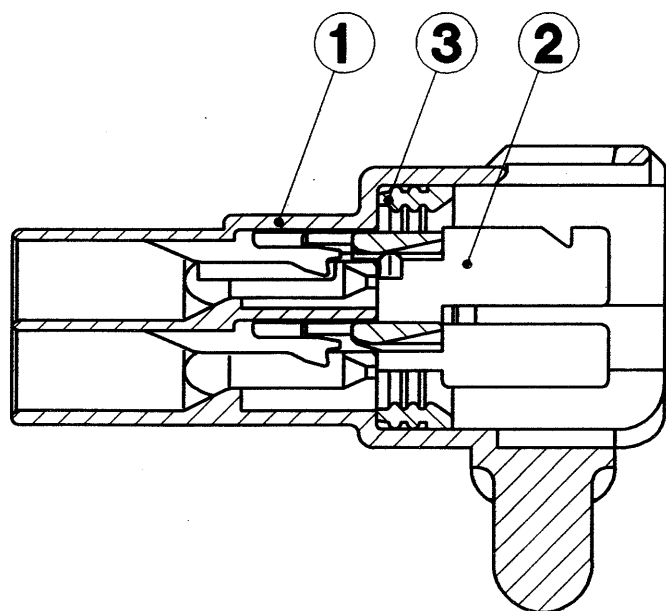
SEC. A-A
